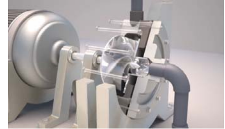
ウォータポンプ 水流の表現
