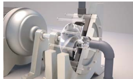
ウォーターポンプ 水流の表現
